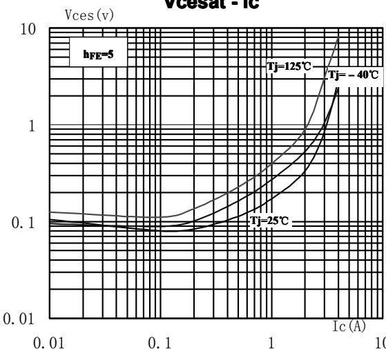
V_{cesat} - I_c
